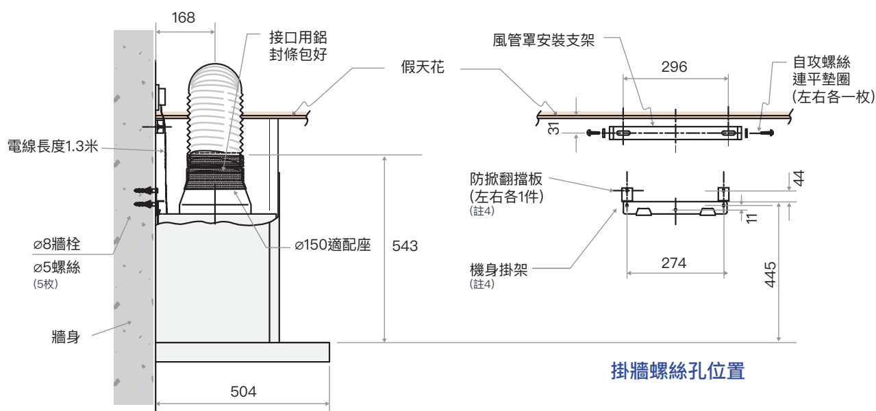
側視圖
