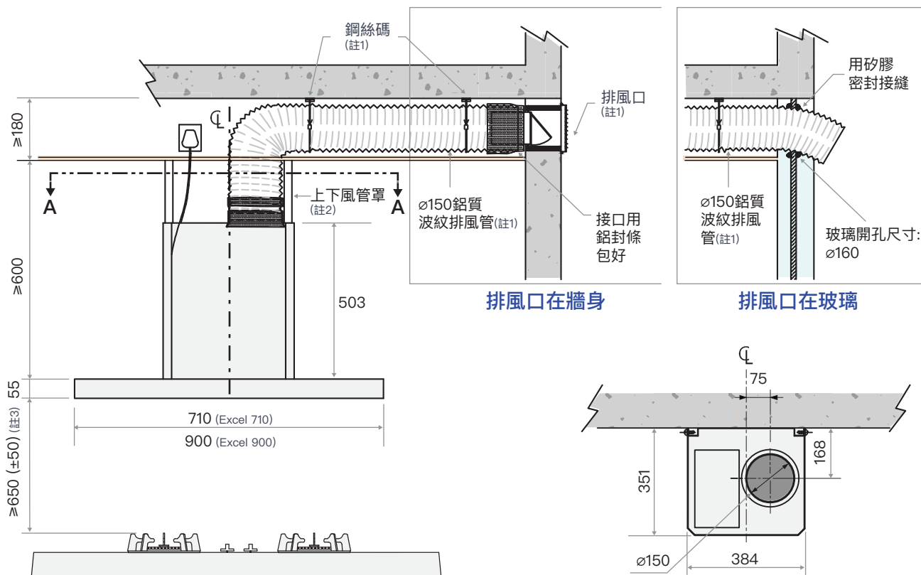
正視圖
